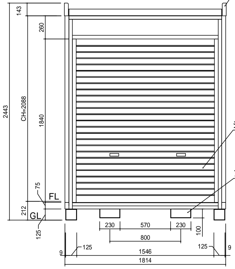
C側立面図 1/25
