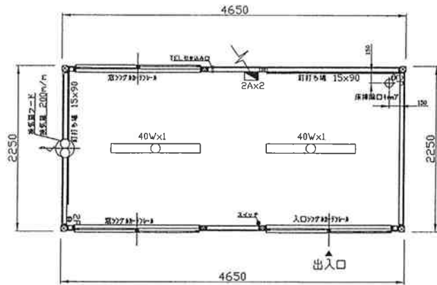
単棟平屋平面図
