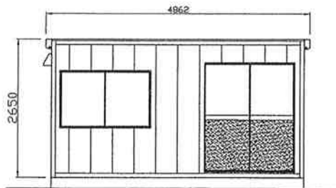
A側立面図
