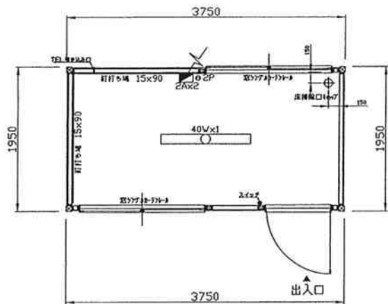
単棟平屋平面図
