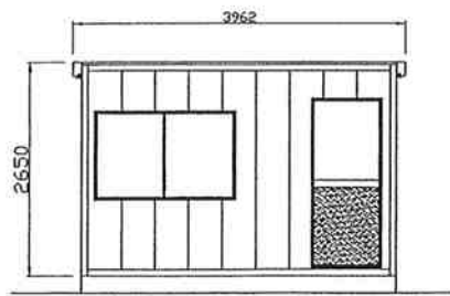
A側立面図
