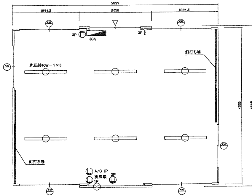
SP-3WR
