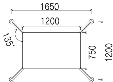
<アウトリガー張出状態図>
