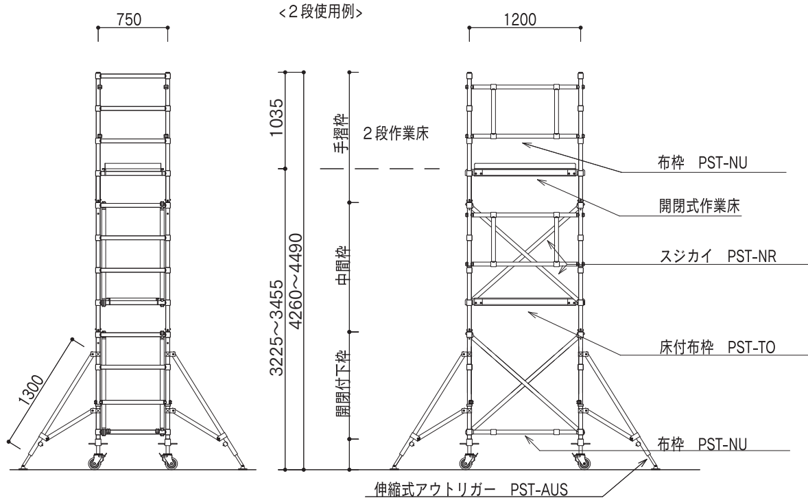
<アウトリガー張出状態図>
