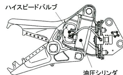
油圧シリンダ
